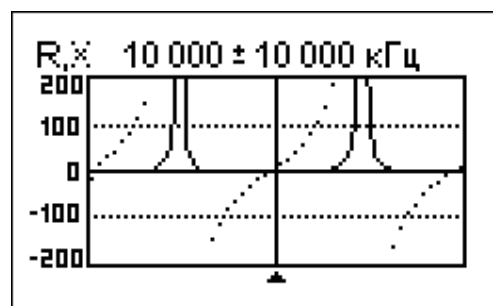
Короткозамкнутый кабель
