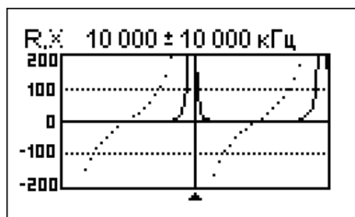
Разомкнутый кабель
